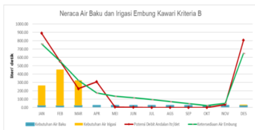
Gambar 7. Neraca air embung kawari kriteria B
