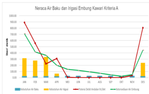
Gambar 6. Neraca air embung kawari kriteria A
