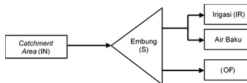
Gambar 2. Skema aliran rencana embung kawari
