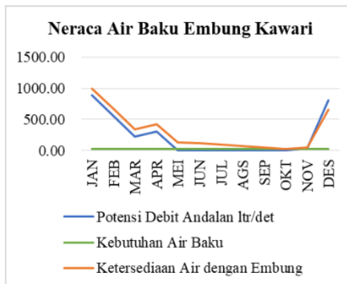
Gambar 5. Neraca air baku embung kawari
